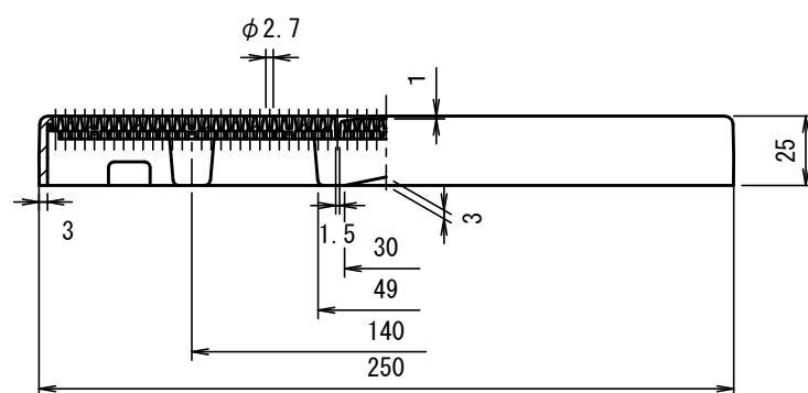
B-B断面図
